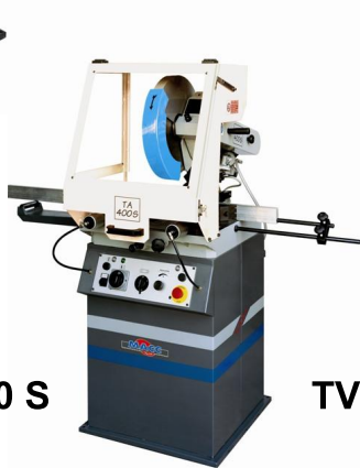
TA 400 - terä kallistuu 45° vas.
